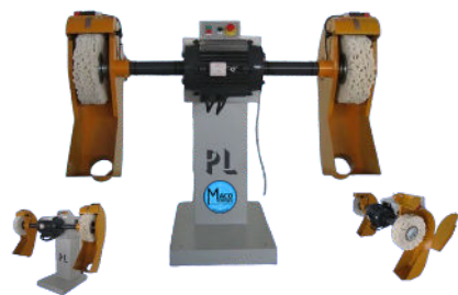
TOURET À POLIR
